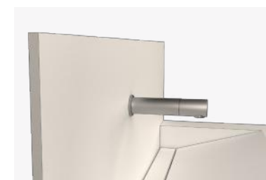
SANS PLAGE (M) Mitigeur mural sans accès. Dimensions de la crédence : 300mm x 12mm. Dans cette configuration, le plan fait seulement 450 mm de profondeur (PMR).
