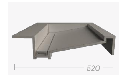
JLB Idem que le style JB "stop goutte". Intérieur: (sur mesure) x350x80mm
