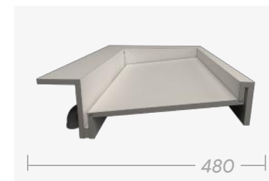
JLT Idem que le style JT "stop goutte". Intérieur: (sur mesure) x350x80mm
