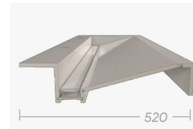
JB Cache caniveau amovible pour entretien. Intérieur: (sur mesure) x350x80mm
